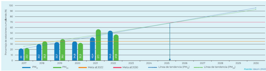
Figura 6. Evaluación anual del porcentaje de estaciones de monitoreo de la calidad del aire en Colombia que cumplen con el “Objetivo Intermedio 3 de la OMS” para PM10 y PM2,5
