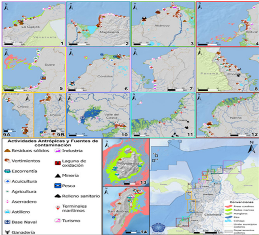
Figura 5. Principales fuentes de contaminación en la zona marino4costera de Colombia
