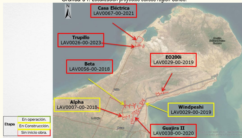
Gráfica 94: Localización proyectos eólicos región Caribe.
