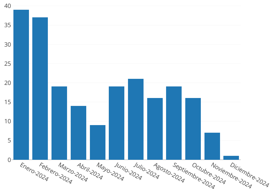
Número procesos
