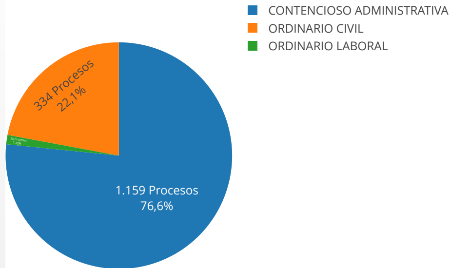
Número procesos
