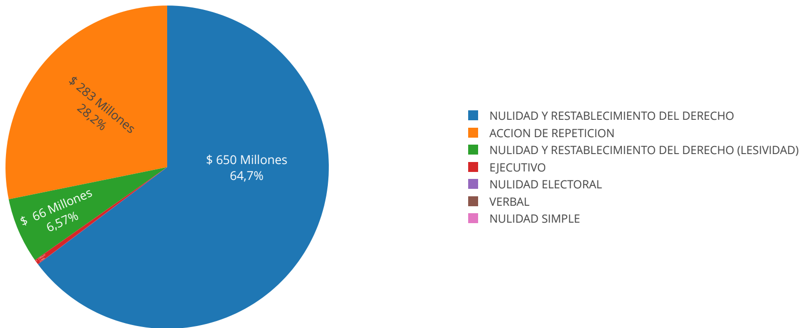
Pretensiones
