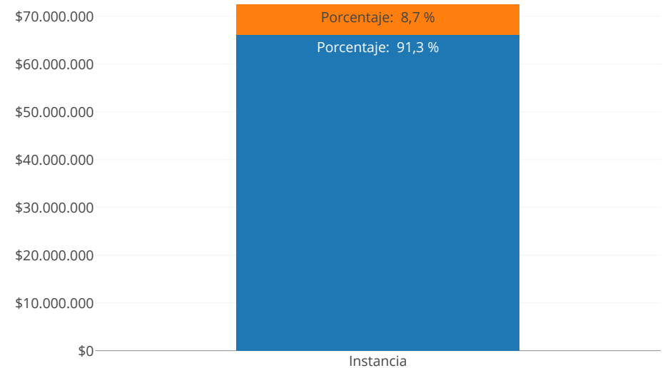
Pretensiones (Millones)
