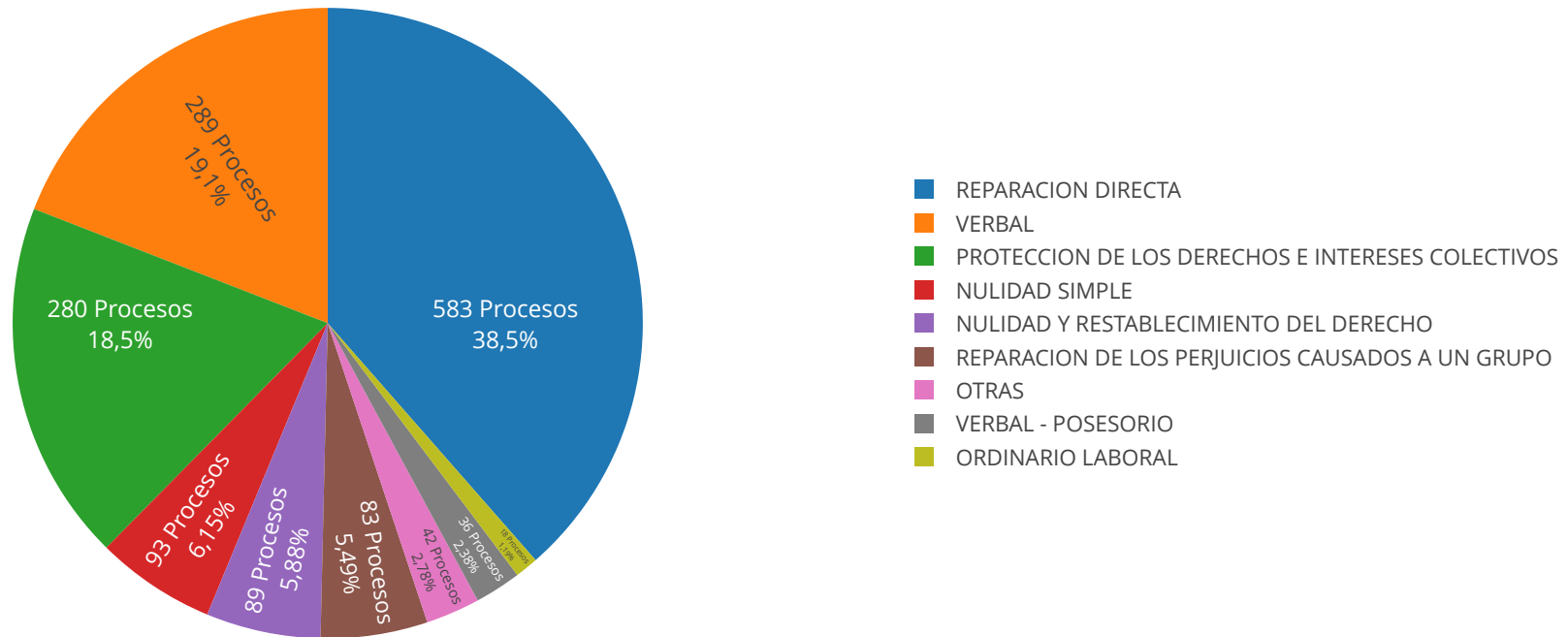
Número procesos
