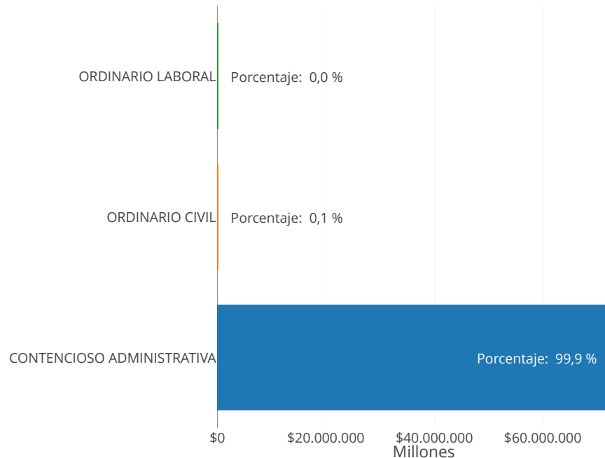
Pretensiones (Millones)
