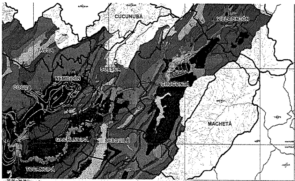
Figura 2. Unidades de importancia hidrogeológica relacionadas con el área solicitada en sustracción.
