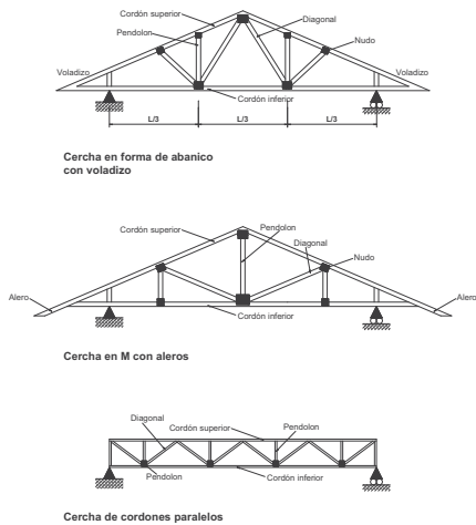
Figura G.8.1-1 — Elementos en armaduras comunes
