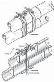
Figura G.12.11-4 - Zunchos
