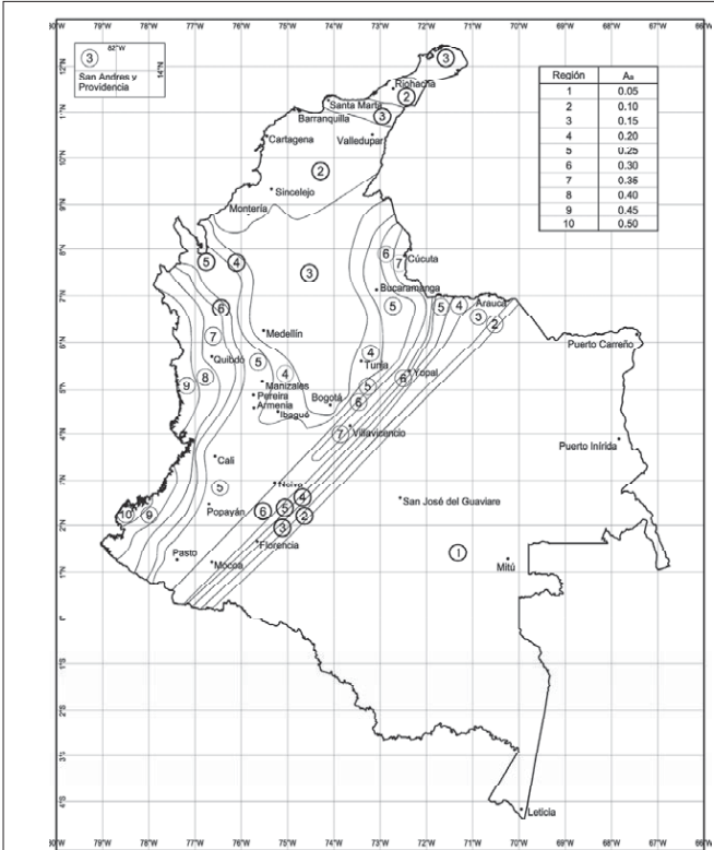
Figura A.2.3-2 — Mapa de valores de A_s
