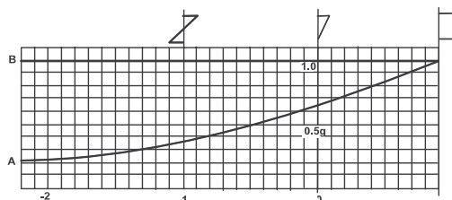
Figura F.5.4.3-2 — Elementos planos bajo gradiente de esfuerzos, valor de g
