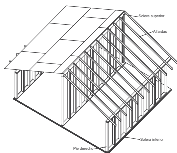
Figura G.9.3-1 — Sistema de entramado liviano
