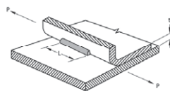
Figura F.4.5.2-13 — Cortante en soldadura abocinada en media V
