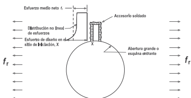
(b) concentrador de gran esfuerzo (abertura grande)
