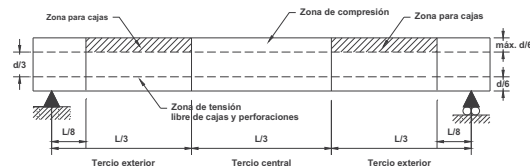
Figura G.3.4-2 — Indicaciones para cajas
