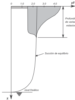
Figura H.9.4-1 — Variación estacional de la succión en relación con la profundidad
