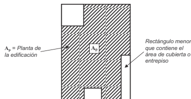
Figura E.7.8-1 — Descripción del rectángulo menor que contiene el área de la cubierta o entrapiso
