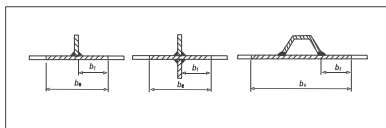
Figura F.5.5.4-4 — Sección efectiva de rigidizador
