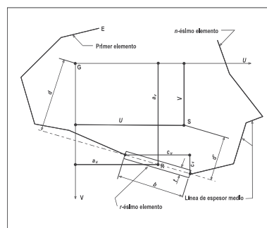
Figura F.5.F-5 — Notación de sección asimétrica
