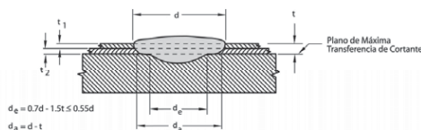
Figura F.4.5.2-6 — Soldadura de tapón — Doble espesor de lámina
