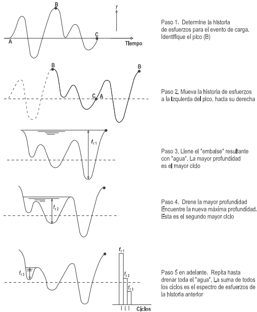
Figura F.5.7.7-1 — Método del embalse para el conteo de ciclos
