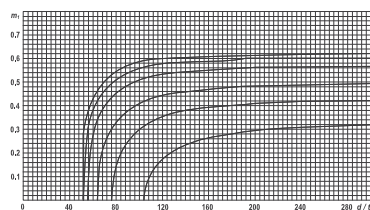
Figura F.5.5.4-3 — Coeficiente de pandeo por cortante m_1
