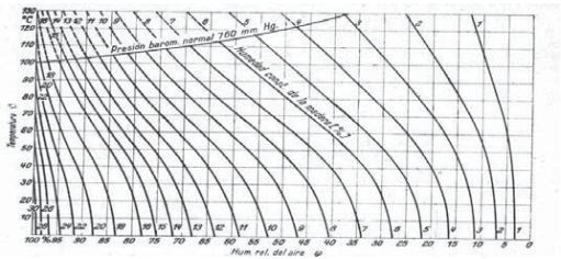
Figura G-D.1 — Isotermas de Sorción
