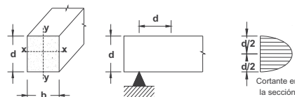
Figura G.3.4-1 — Esfuerzo Cortante en vigas.
