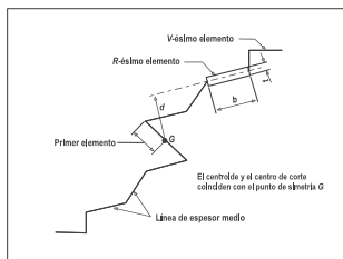
Figura F.5.F-4 — Notación de sección con simetría oblicua
