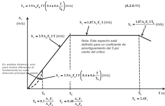
Figura A.2.6-2 — Espectro Elástico de Velocidades (m/s) de Diseño
