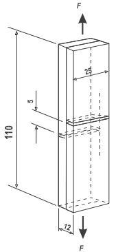
Figura F.5.6.10-1 — Ensayo de corte con capa gruesa de adhesivo
