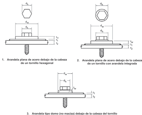
Figura F.4.5.4-1 — Desgarramiento del material en contacto con la arandela
