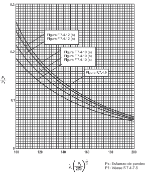
Figura F.5.1-1 — Resistencia al pandeo con alta esbeltez
