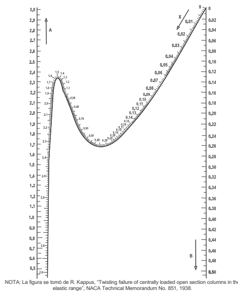
Figura F.5.H-4 — Nomograma para resolver la ecuación cúbica x^3 - 3x^2 + Ax - B = 0
