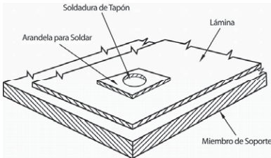
Figura F.4.5.2-1 — Arandela para soldadura típica
