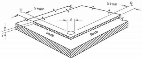
Figura F.4.5.2-3 — Distancia al borde para soldaduras de tapón — lámina sencilla
