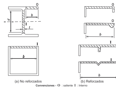
Figura F.5.4.3-1 — Tipos de elementos planos
