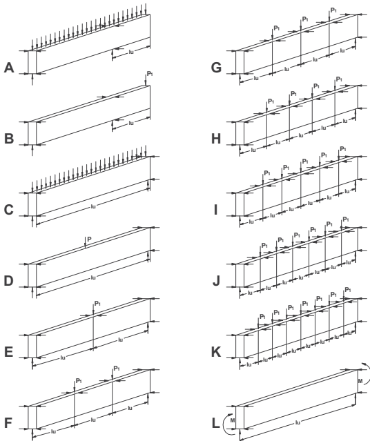
Figura G.3.3.2 — Casos escogidos de cargas y soportes laterales. Véase tabla G.3.3-4 (Referencia RG.9)
