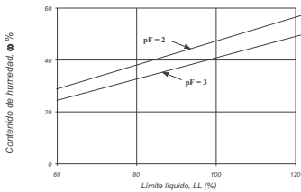
Figura H.9.4-2 — El contenido de humedad como expresión de la succión para diferentes tipos de suelos representados por el límite líquido
