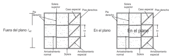
Figura G.4.3-1 — Arriostramiento de entramados
