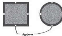
Figura J.3.5-1 — Perforaciones de las secciones de acero huecas rellenas de concreto.
