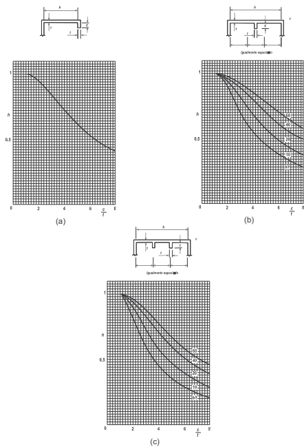
Figura F.5.4.3-4 — Elementos reforzados, valor de \beta (c) Elementos curvos internos — En elementos curvos de poca altura sometidos a compresión uniforme, \beta debe determinarse usando:
