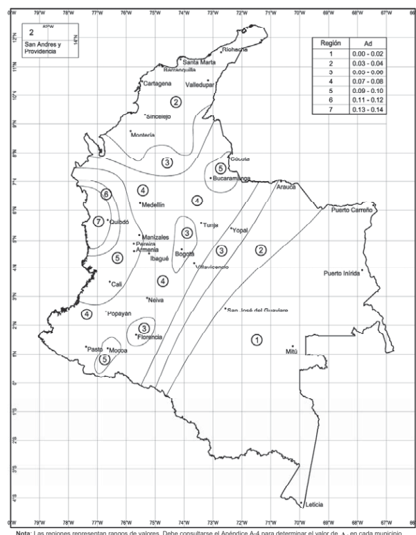
Figura A.12.2-1 — Mapa de valores de A_d
