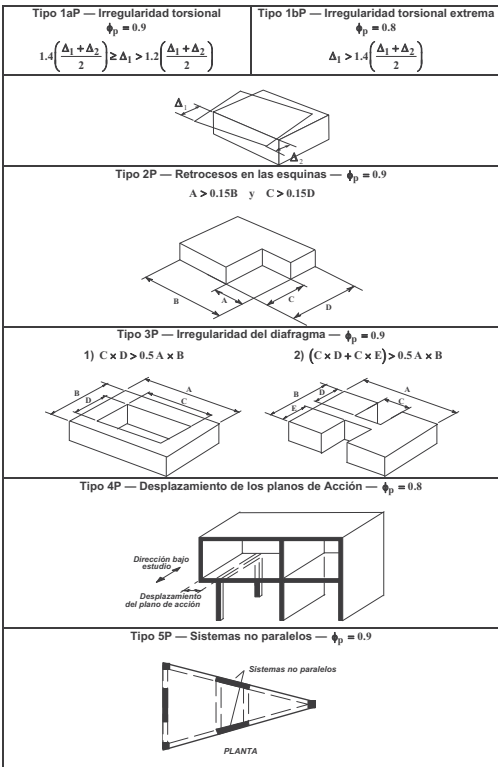
Figura A.3-1 — Irregularidades en planta
