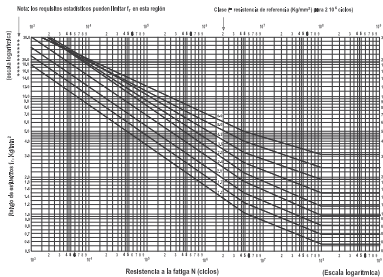
Figura F.5.7.7-4 — Curvas f_r - N de diseño (para historias de esfuerzos de amplitud variable)
