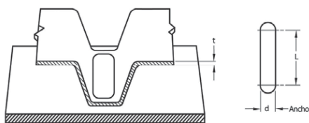
Figura F.4.5.2-8 — Soldadura de ranura — Lámina a miembro de soporte posición plana
