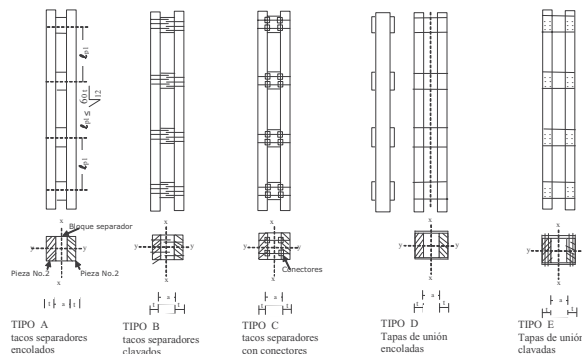
Figura G.4.3-3 — Columnas compuestas espaciadas
