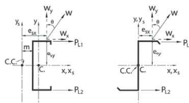
Figura F.4.4.3-1 — Sistema de coordenadas y direcciones positivas de las fuerzas
