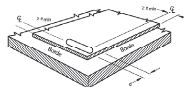
Figura F.4.5.2-9 — Distancias al borde para soldadura de ranura
