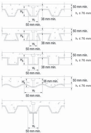
Figura F.2.9.3-1 Límites dimensionales para vigas compuestas con tablero metálico
