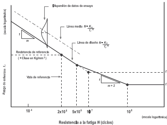
Figura F.5.7.7-3 — Relación f_r - N típica
