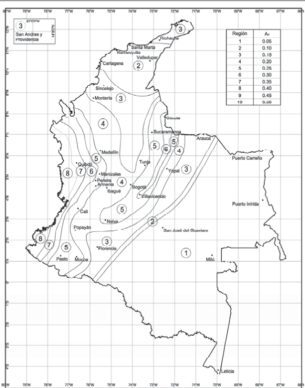
Figura A.2.3-3 - Mapa de valores de A_v
