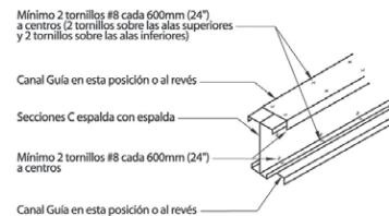
Figura F.4.8.4-5 — Dintel tipo espalda con espalda
