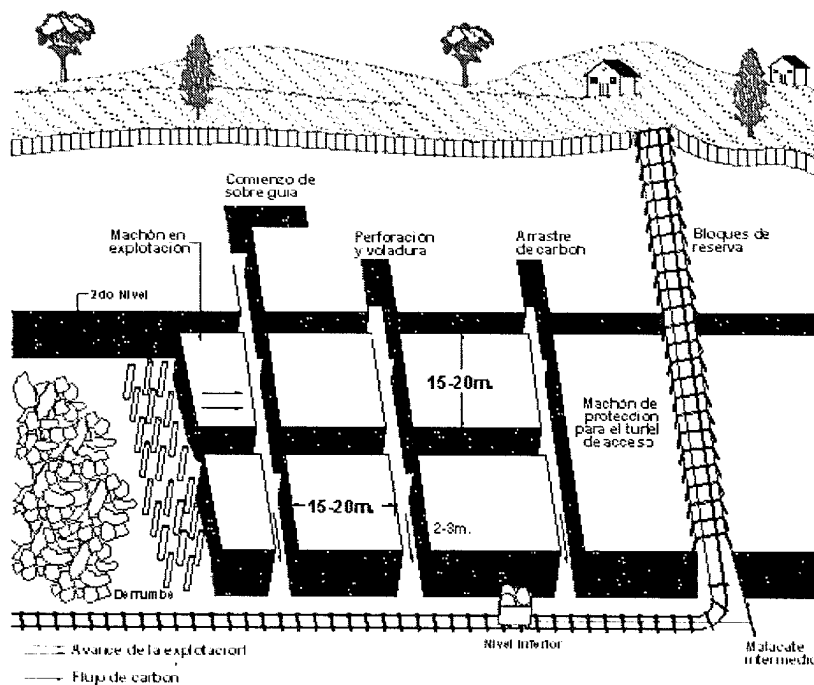
Hundimiento por cámaras y pilares FUENTE: ECOCARBÓN
