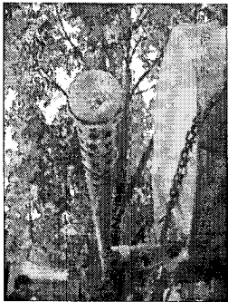
Detalle de la tubería ranurada – Flauta para irrigación FUENTE: PMA, para la fase de operación de la termoeléctrica “EL REMANSO” – TERMOPAIPA IV 2004
