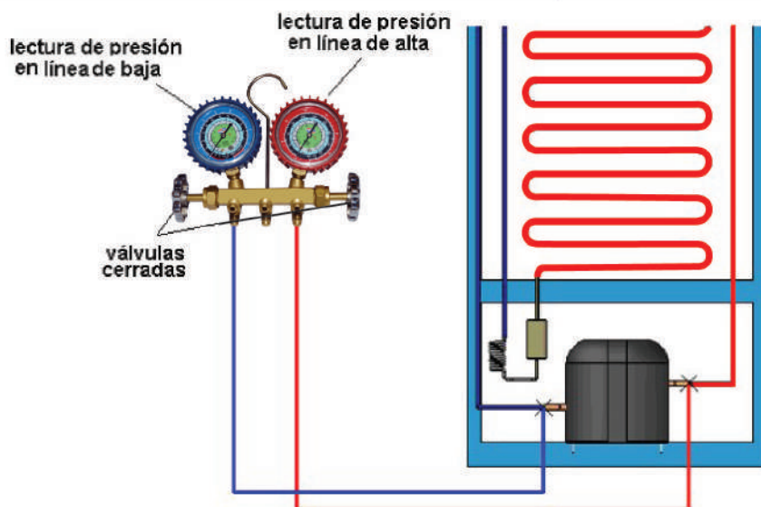
Figura 20. Conexión del árbol de manómetros a línea de alta presión y línea de baja presión
