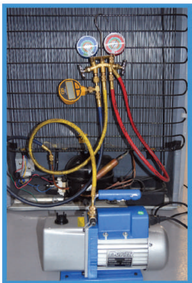
Figura 58. Conexión de la bomba de vacío al sistema
