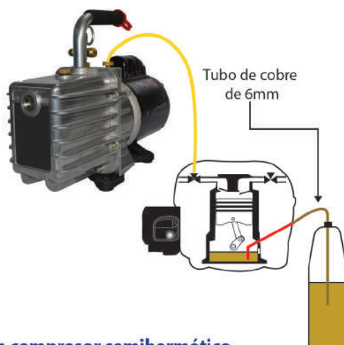
Figura 39. Llenado de aceite en compresor semihermético
