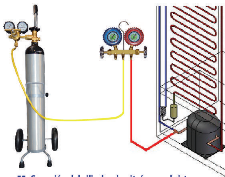
Figura 55. Conexión del cilindro de nitrógeno al sistema
