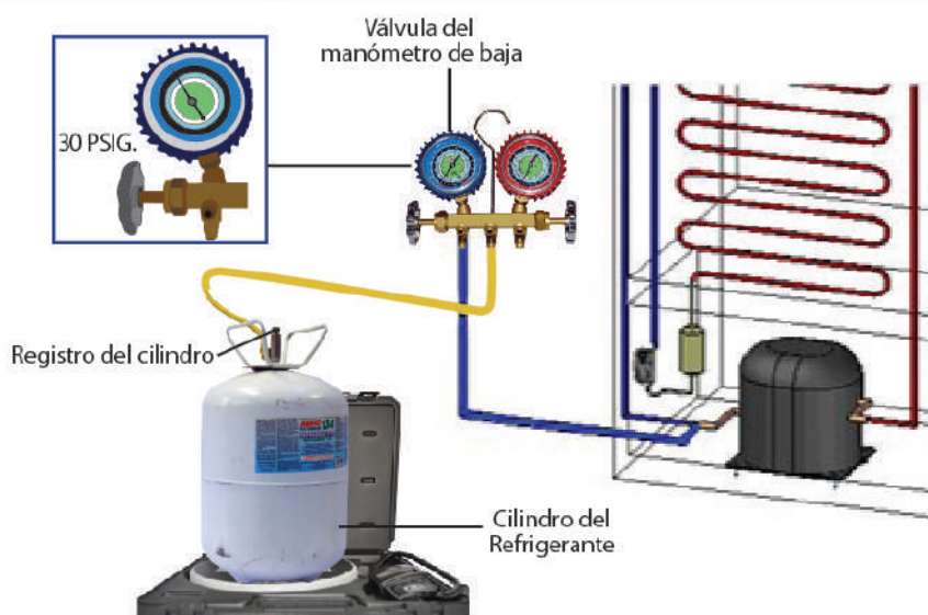
Figura 63. Ejecución de la precarga
