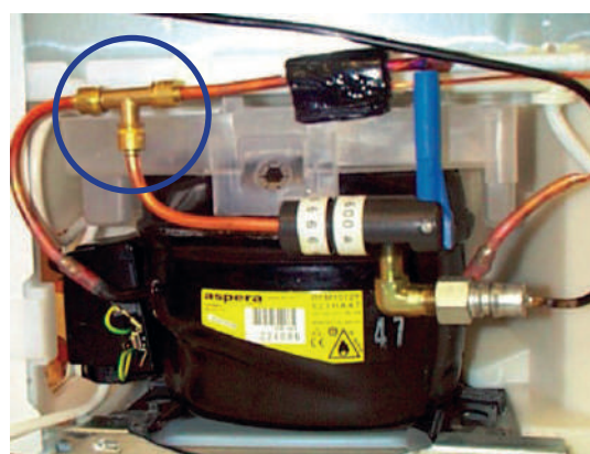
Figura 54. Ejemplos de uniones con unión en frío o tipo Lokring en T
