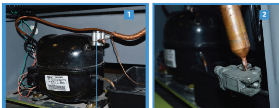
Válvula pinchatubo
