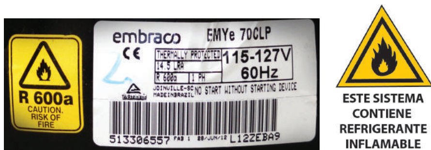
Figura 69. Etiquetas para rotulado con hidrocarburos HC
