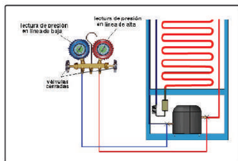
Figura 21. Verificación de presión de estabilización
