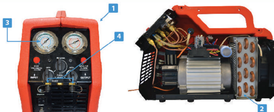
Figura 29. Ejemplo de recuperadora adecuada
