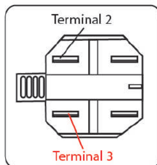
Figura 17. Relé electromecánico tipo "EG y PTC"
