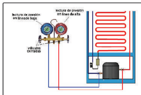
Figura 22. Verificación de presiones y temperaturas de trabajo
