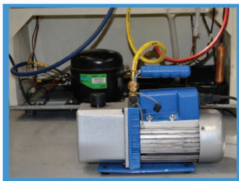
Figura 58. Conexión de la bomba de vacío al sistema
