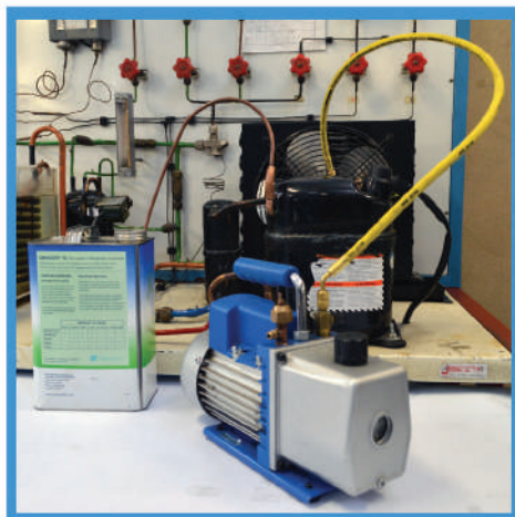
Figura 39. Llenado de aceite en compresor semihermético
