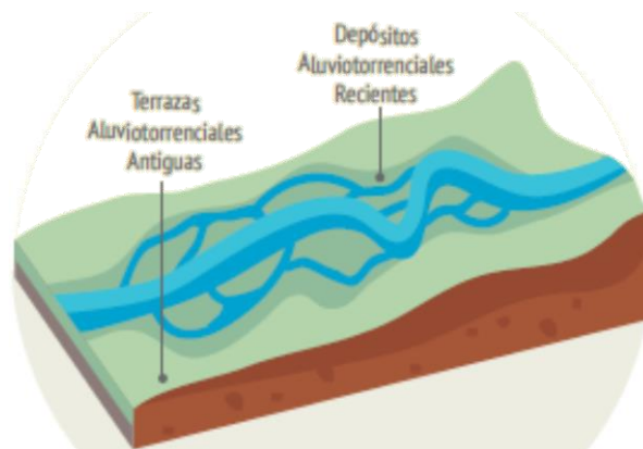
Figura 2-14. Esquematización de un río trenzado.
