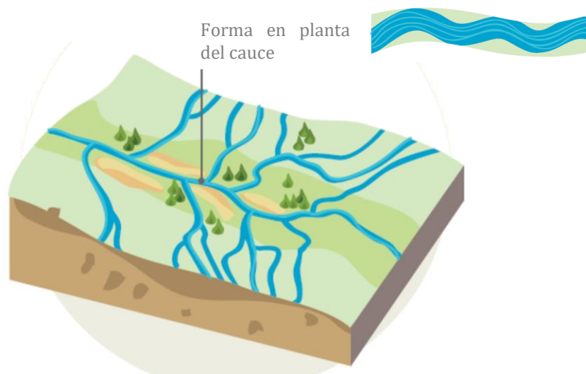
Figura 2-10. Esquematación de un río recto de montaña con su forma típica en planta.
