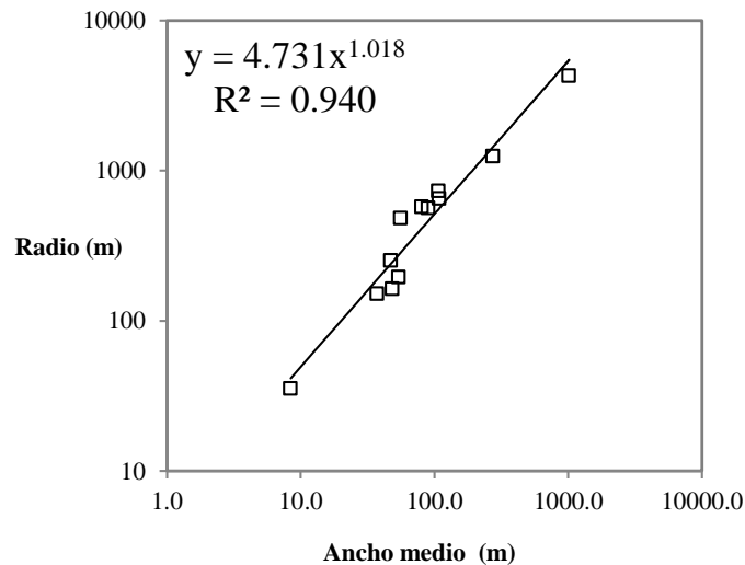
Figura 6-2. Relación de invarianza para el radio de curvatura R_c .
