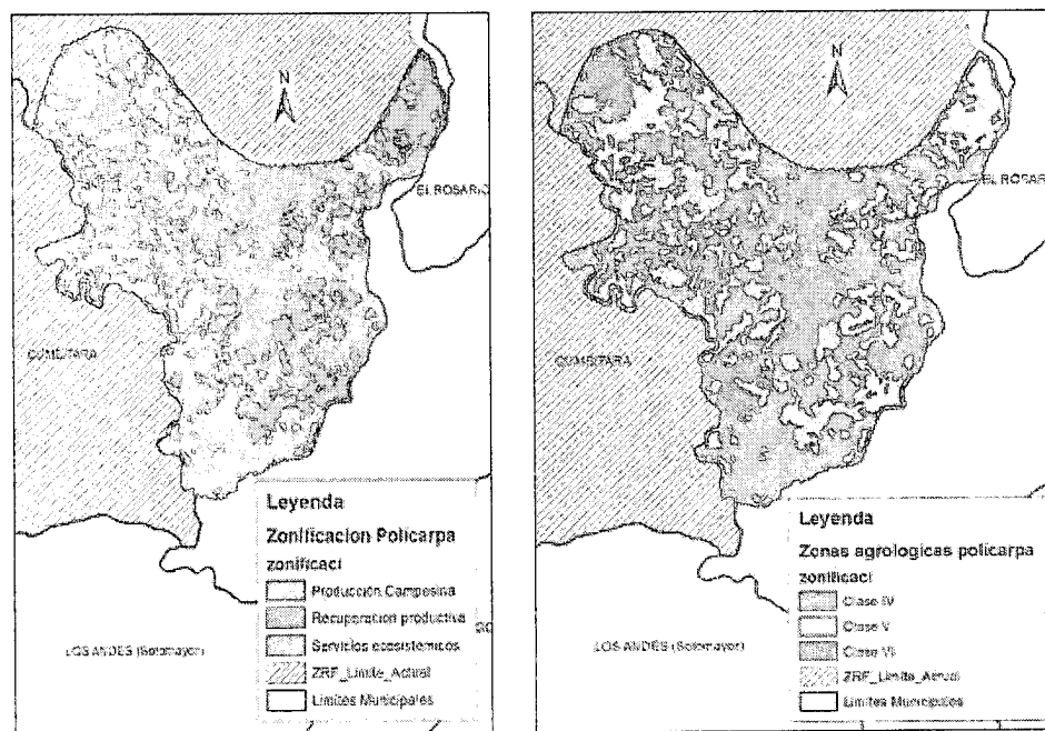
Figura 1. Izquierda: Zonificación ambiental municipio de Policarpa. Derecha: clases agrológicas municipio de Policarpa.
