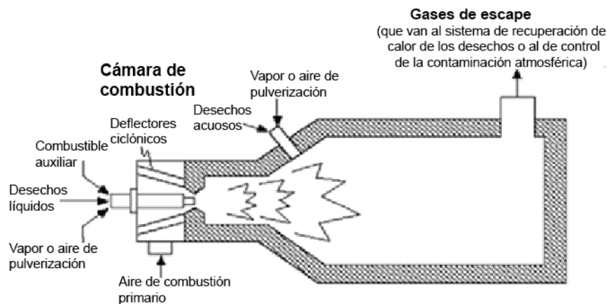
Figura 3 Incinerador por inyección de líquido
