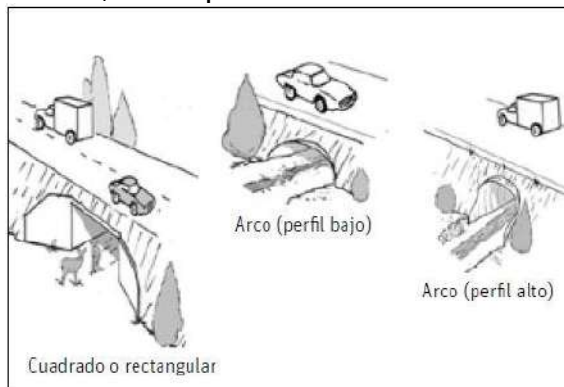
Figura 38: Opciones de diseño de Box-culvert, como pasos de fauna.
