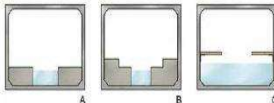
Figura 37_: Secciones transversales de Box culverts con pasos de fauna.
